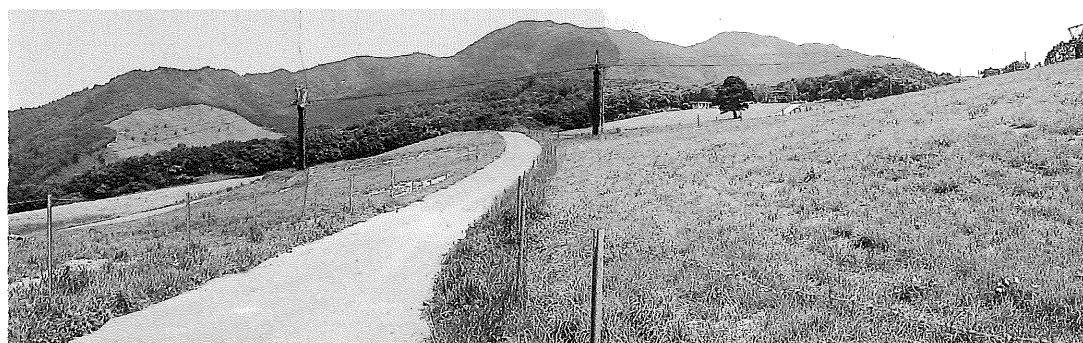
写真一 4 天童高原の古い地すべりによる緩斜面と面白山
