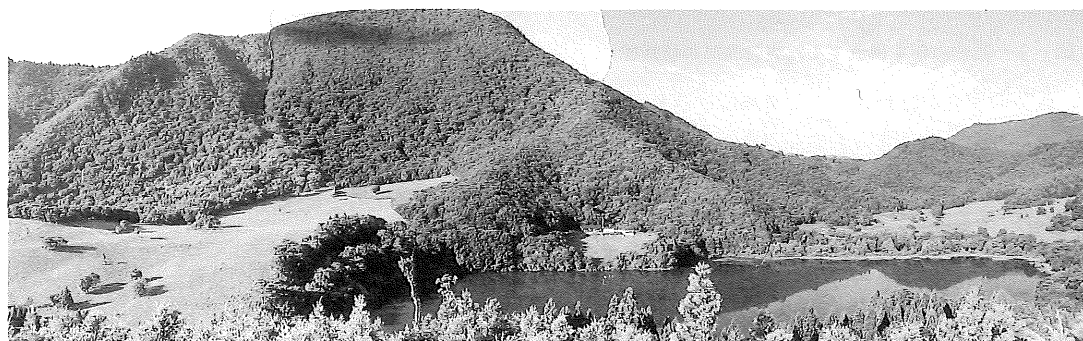
写真一 3 堂木沢山の地すべり斜面と、そのせき止めによって生じた沼沢沼
