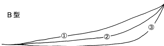
図一六 侵食の進行の2つの様式 ①～③は順に各段階を表わす。隆起量は③段階のものに合わせた A型：崩壊前線といった激しい侵食が伴って進行 B型：斜面全般にわたり徐々に侵食が進行
