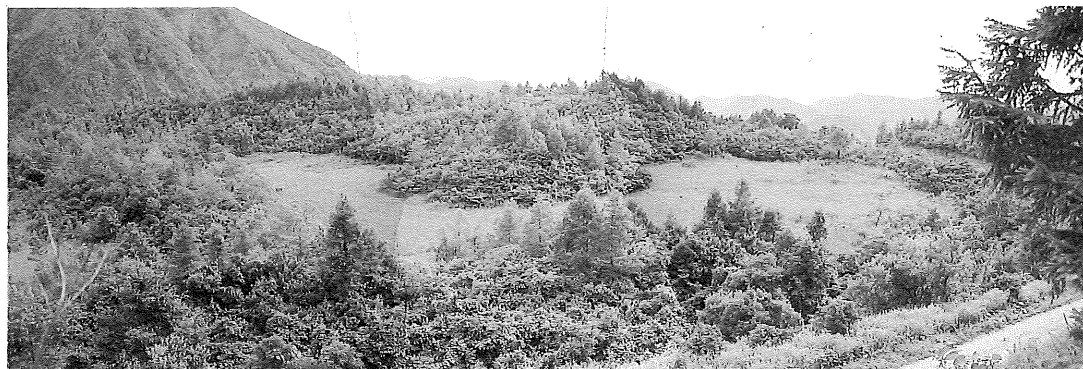
写真一 2 ムクロ沢地すべり滑落土塊の冠頭部を埋める湿地堆積物
