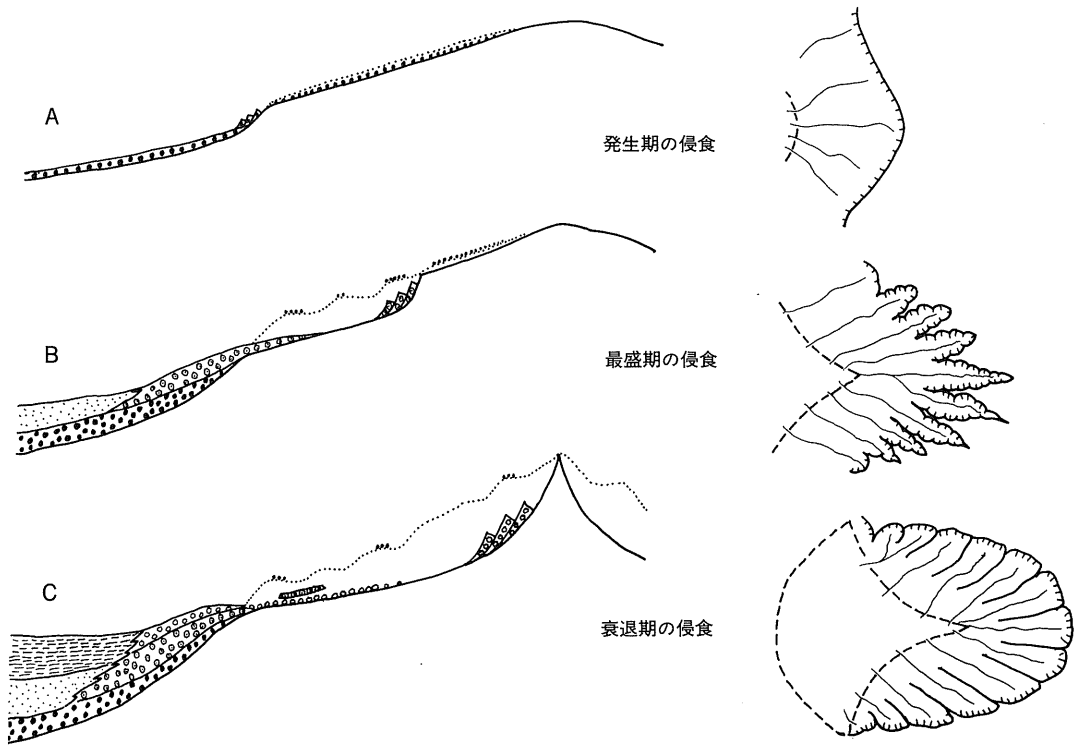
図一五 奥羽山系西斜面の乱川区における侵食過程の変遷模式図
