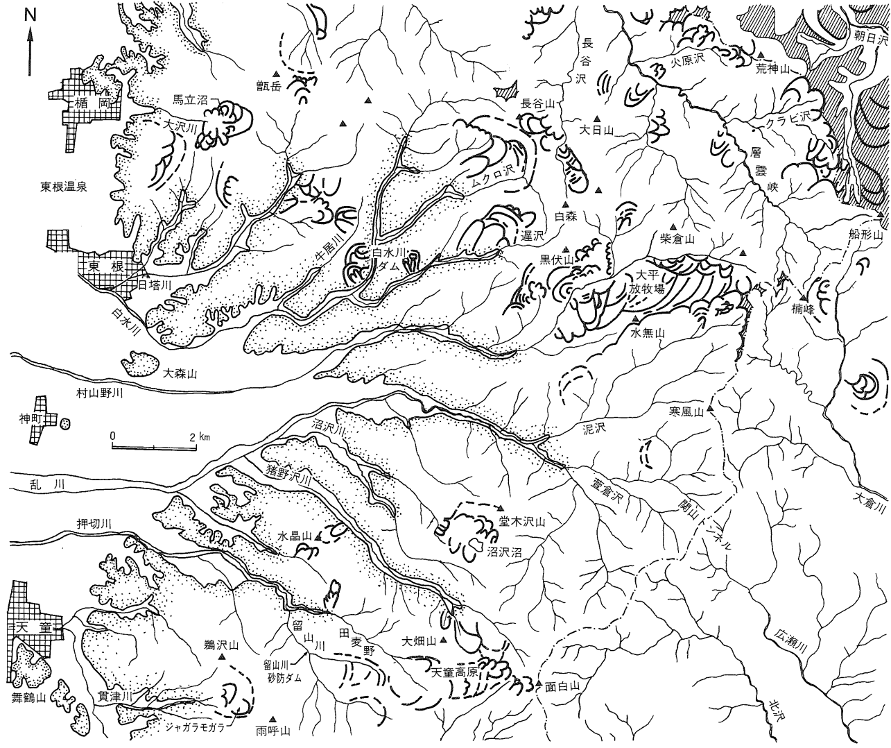
図-1 地すべり地形図
