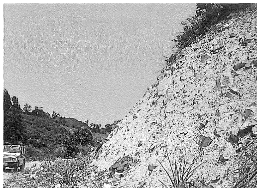
写真一 留山川砂防ダム上流地すべり地内でみられる崩積土塊。凝灰質な砂岩が角礫状に破壊されている。こうした岩質の土塊は地すべり地形の周辺では普通にみられる。
